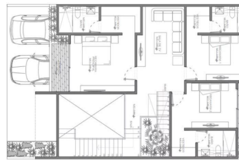
Planta alta
