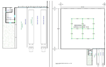
- PLANO ARQUITECTÓNICO-
