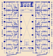
Planta tipo torre norte
