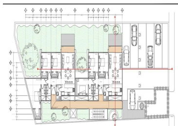
PLANTA ARQUITECTONICA SEÑALADO NIVEL + 3.04
