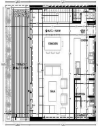
Planta Baja 50 m 2 habitables 21.18 m 2 Terraza
